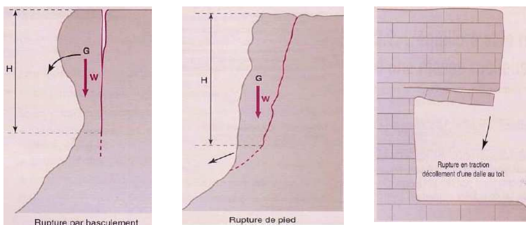
Illustration 3 : schéma de principe des différents types de rupture (basculement, rupture de pied, rupture de surplomb) (source: LCPC et MEDDE)
