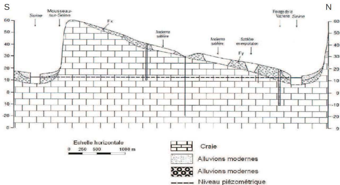
Illustration 2 : coupe géologique selon un axe sud-nord (boucle de Moisson) (source :BRGM)
